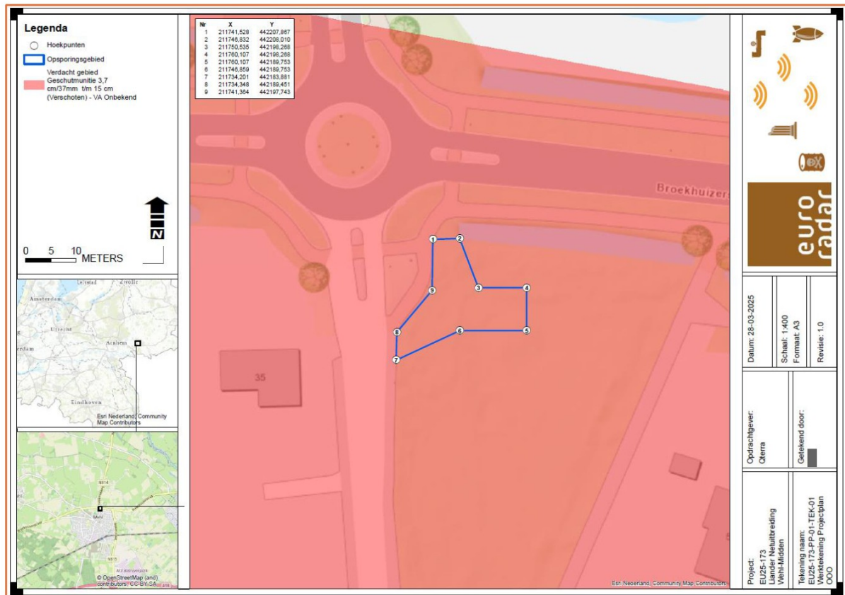
Afbeelding 7: Werktekening EU25-173-PP-01 -TEK-01 (Bron: Euro radar).
